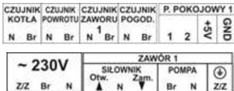
Rys.1. Widok listew przyłączeniowych.
