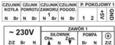
Rys.1. Widok listew przyłączeniowych.
